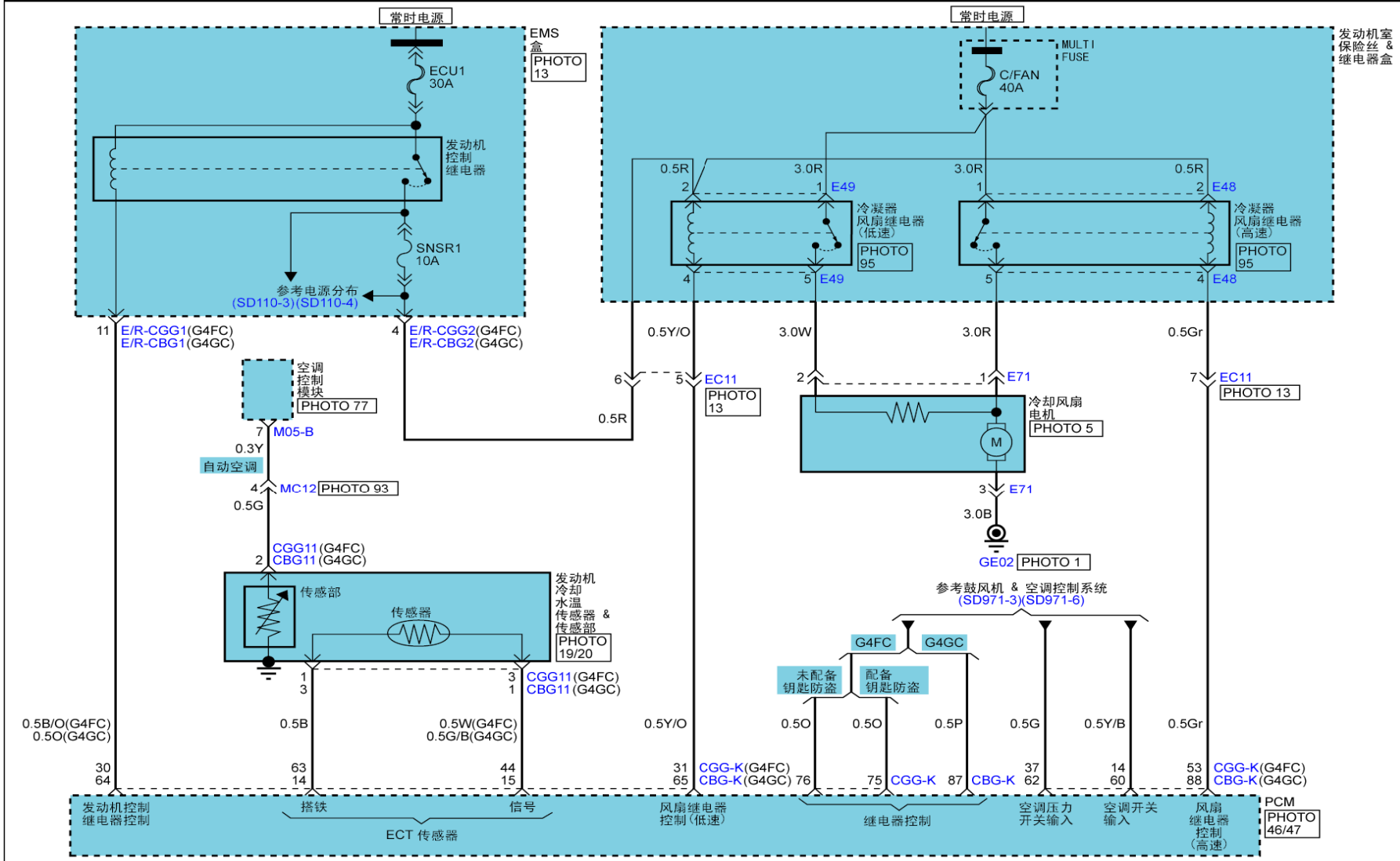
冷却系统 (1)
